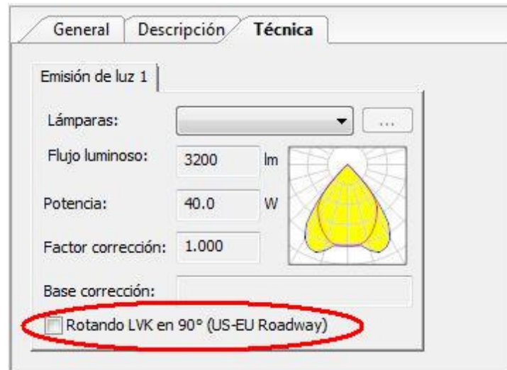
Ilustración 349 Rotación de la curva de distribución de la intensidad luminosa
